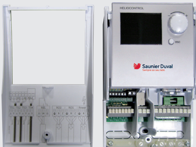
Ligações elétricas
